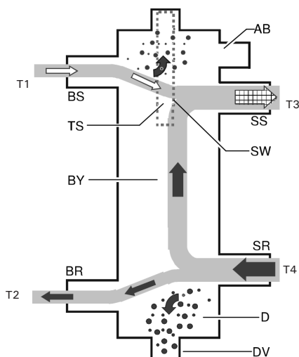
Conception du collecteur à faible perte
