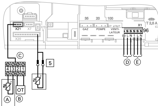
Socle de la boîte de commande de la chaudière
